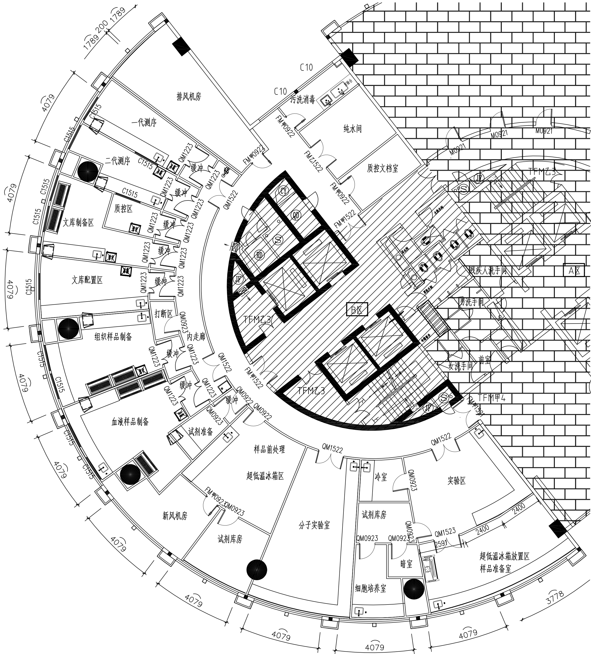
二十一层实验室平面
