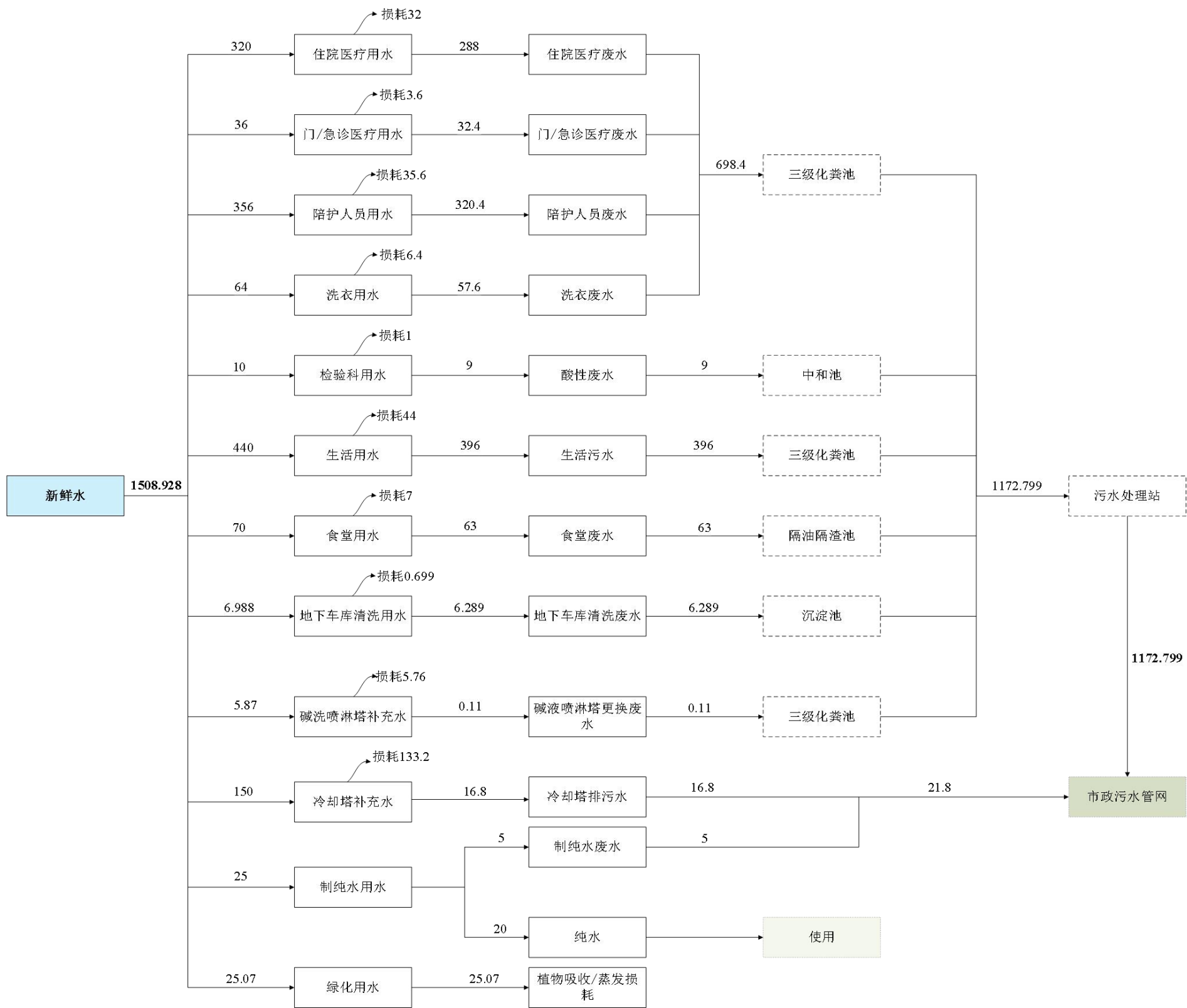
图 2.4-1 水平衡图 单位: m³/d
