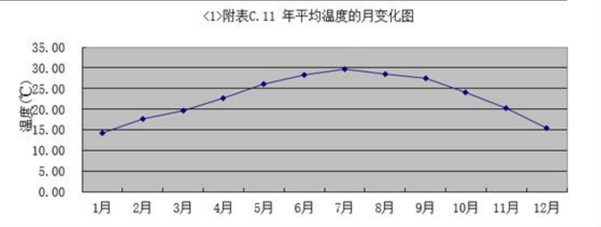
图 5.2-3 广州 2024 年各月平均气温变化图
