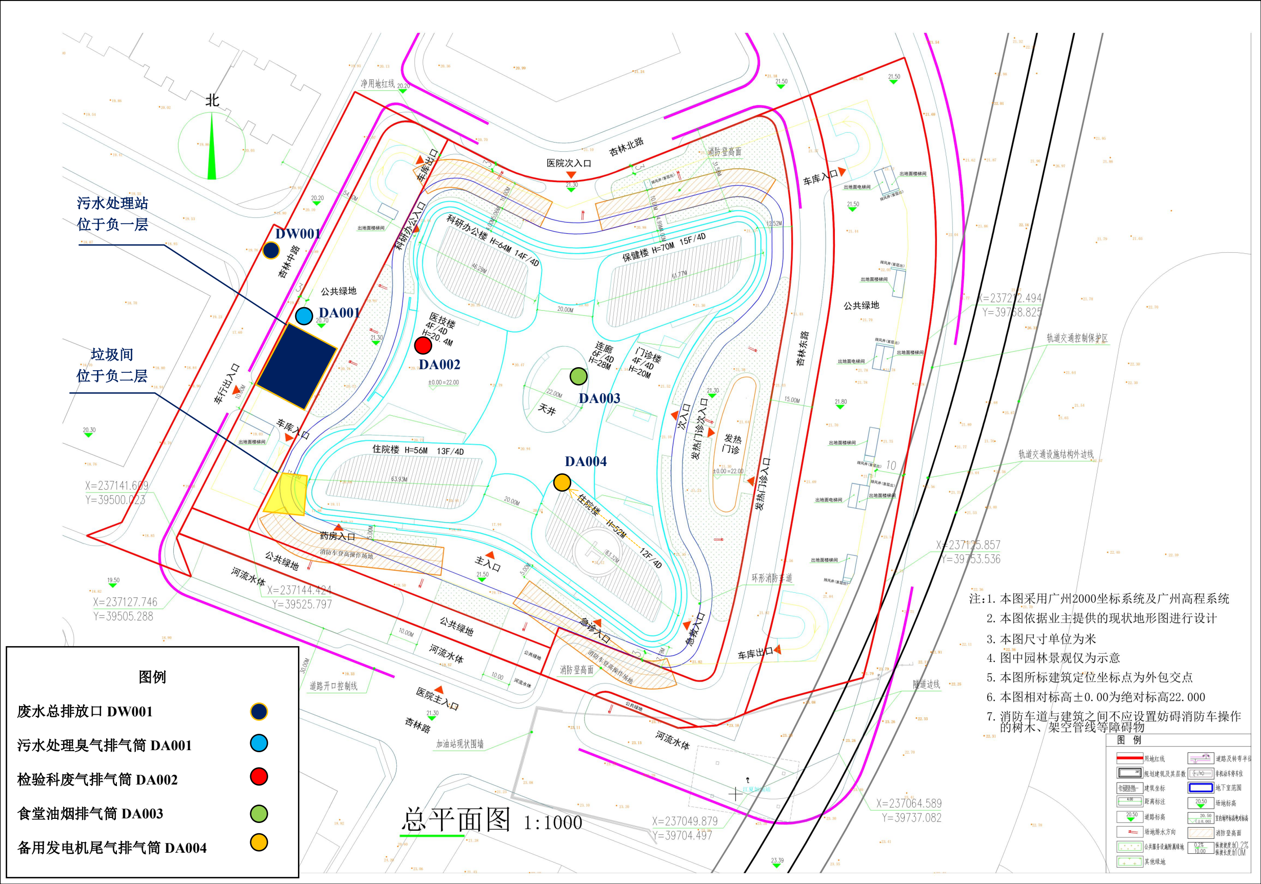
图 2.2-3 环保设施排放口平面布置图
