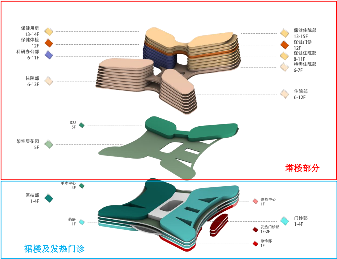
图 2.2-1 功能布局示意图
