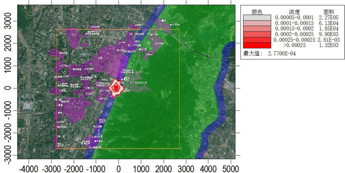
图 5.2-8 硫化氢叠加环境质量现状浓度后 1h 平均质量浓度等值线分布图
