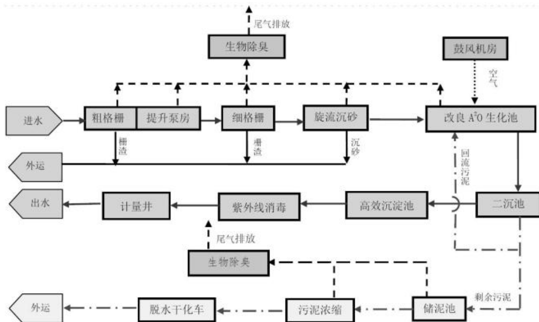
图 5.1-1 污水处理工艺流程图
